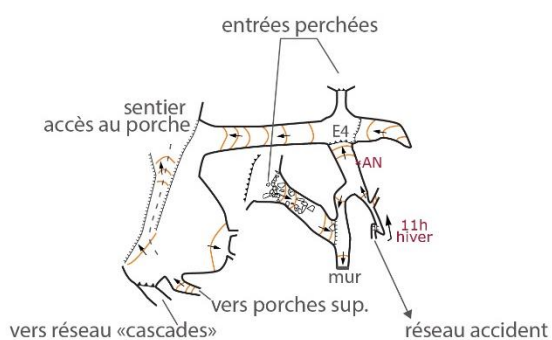
plan schématique de l'entrée «chatière» vers le départ du réseau «accident»
